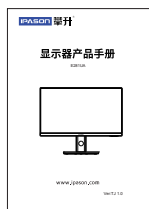
产品手册
